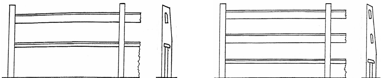
Clôture lissage 1 planche
